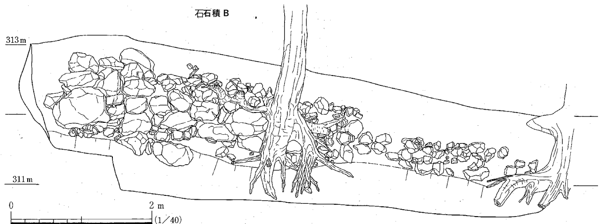
図 60. 石積立面図
