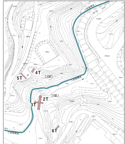
図80. トレンチ位置図
