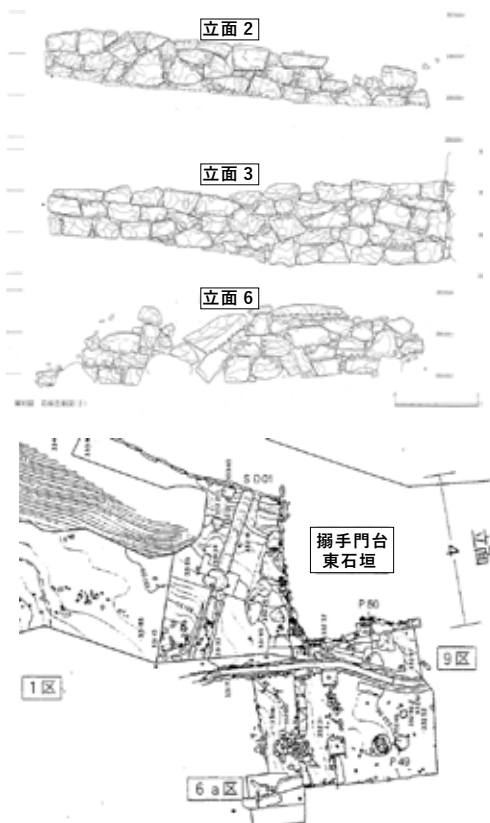
図 45. 搦手門跡周辺および東斜面石垣平面図
