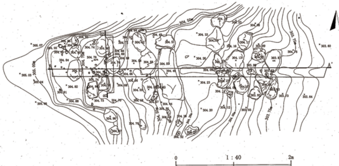
図 63. 城内路跡平面図
