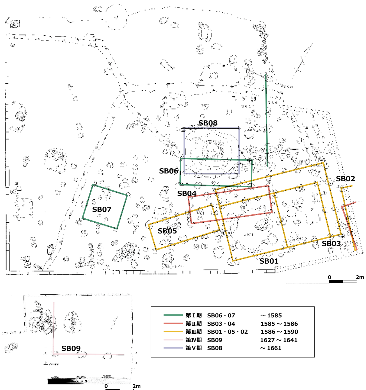
図33. A区およびC－Ⅱ区で検出された遺構
