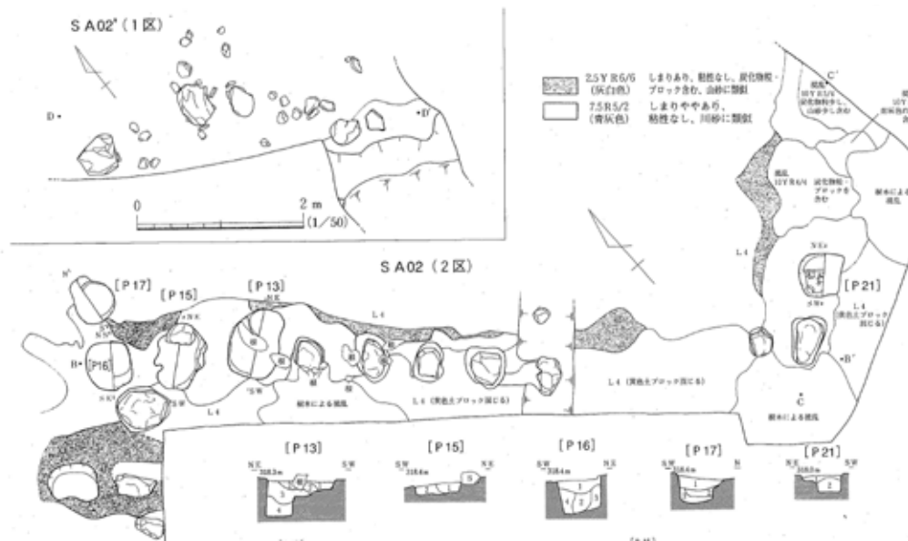
図 54. 屏風折れ礎石立掘立柱塀跡平面図
