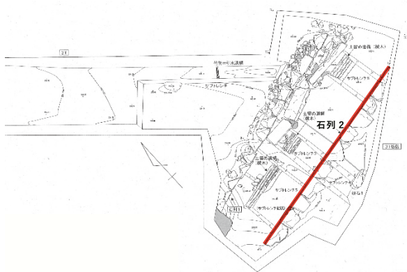
図 130. 調査区平面図
