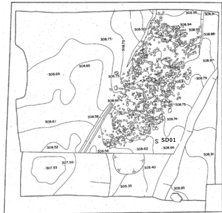
図39. 溝跡平面図
