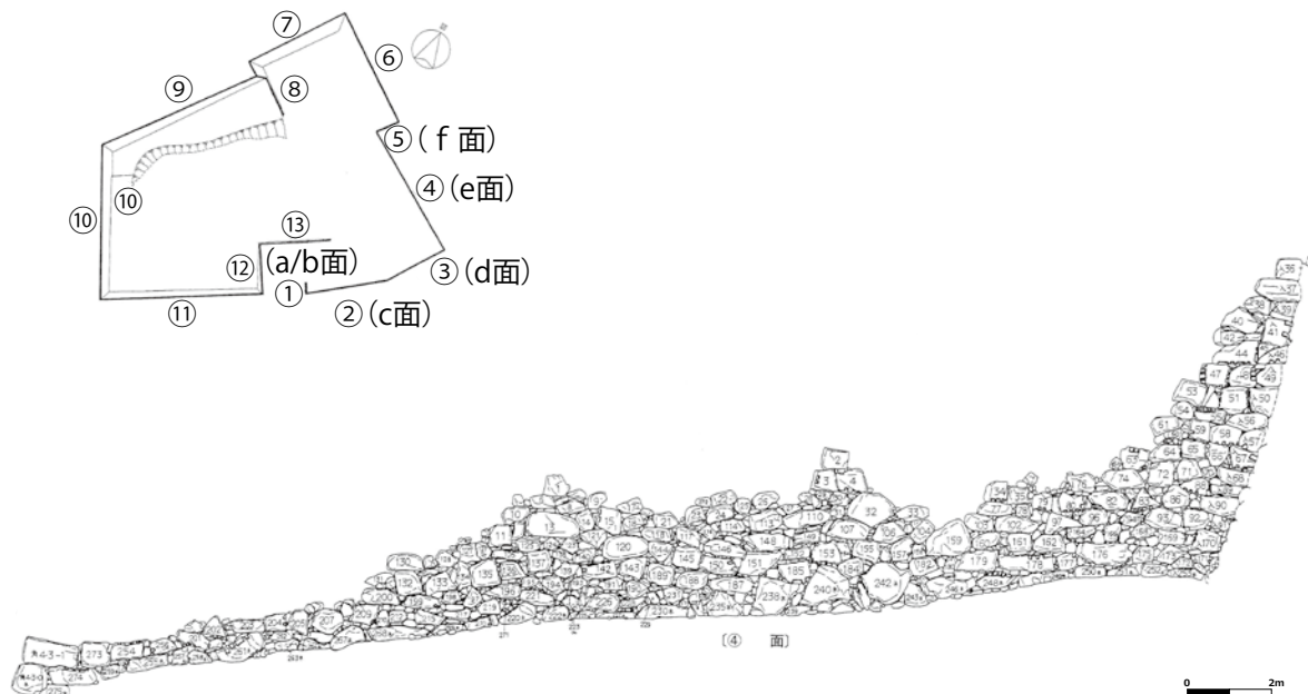
図 35. e 面（④面）の既存石垣立面図
