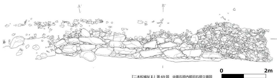
図 36. ⑩面石垣の内部で確認された石垣の立面図
