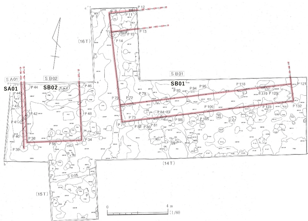
图 77. 14~16T 平面图
