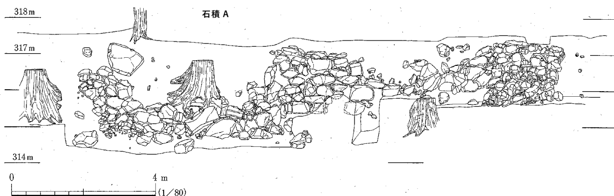
図 59. 石積立面図
