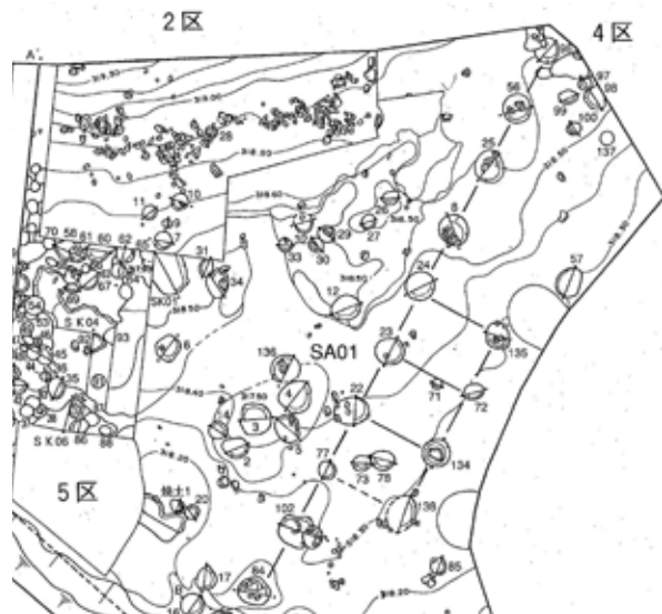
図 53. 掘立柱塀跡平面図
