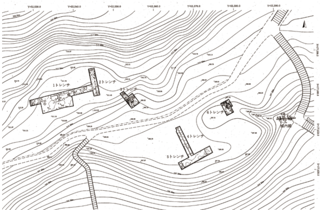
図 62. 大石垣直下の平場 遺構確認平面図
