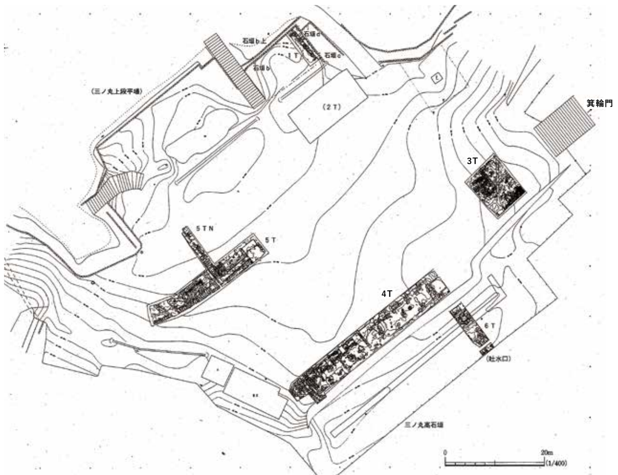
図 88. トレンチ配置図
