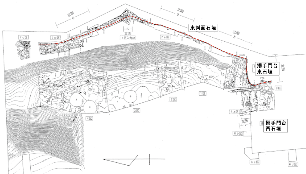
図43. 調査区平面図
