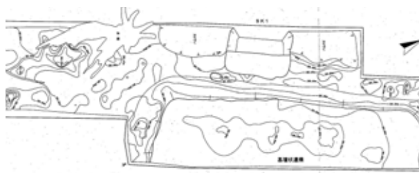
図 111. 1T遺構平面図
