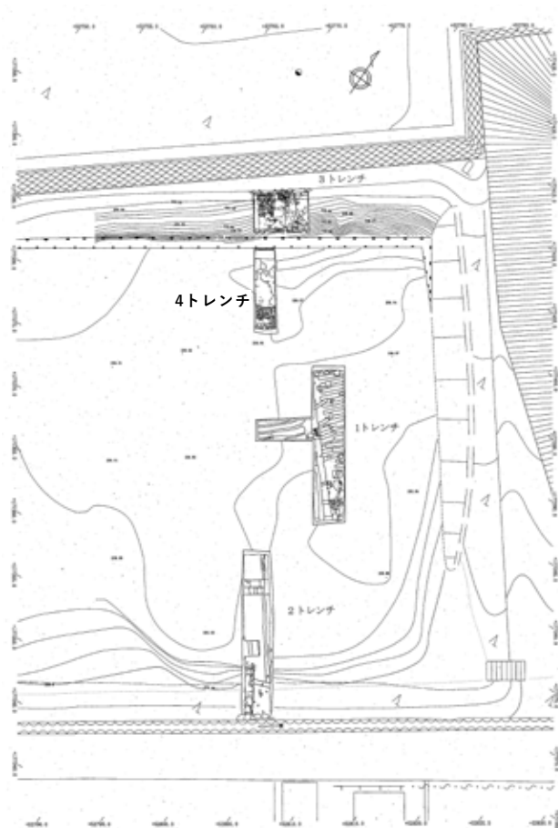
図105. 調査区トレンチ配置図
