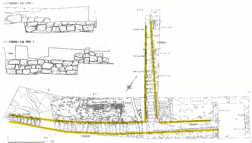
図 90. 5T・5TN遺構配置図
