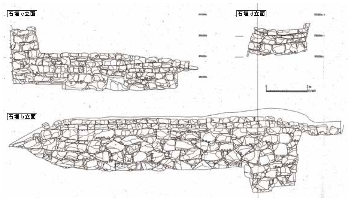
図 94. 石垣立面図(2) 上左: 石垣 c 上右: 石垣 d 下: 石垣 b
