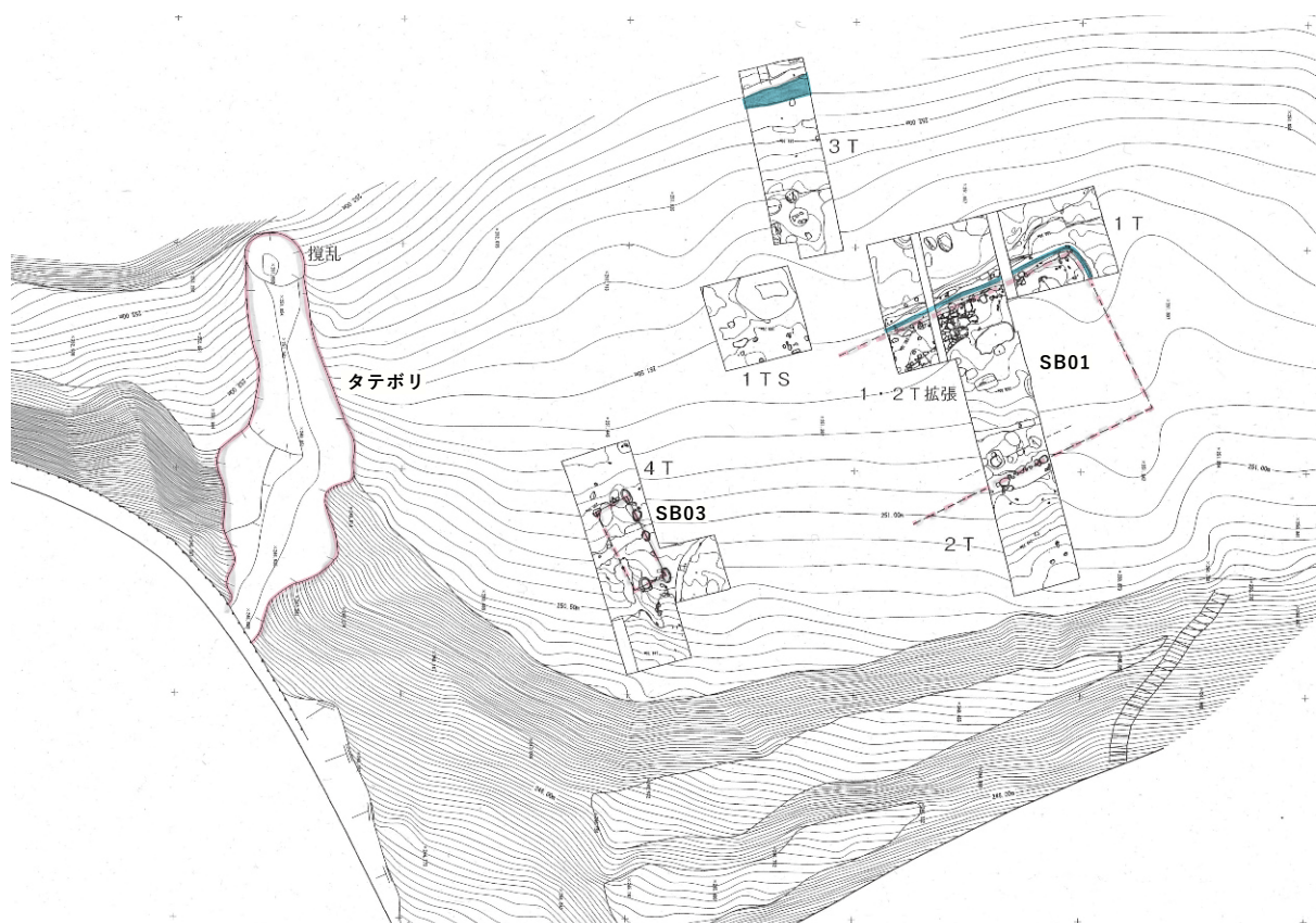
図 119. 調査区トレンチ配置図
